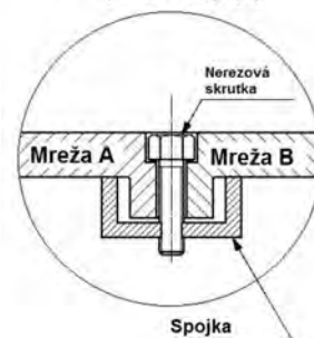
Princíp napojenia mreží pomocou spojky
